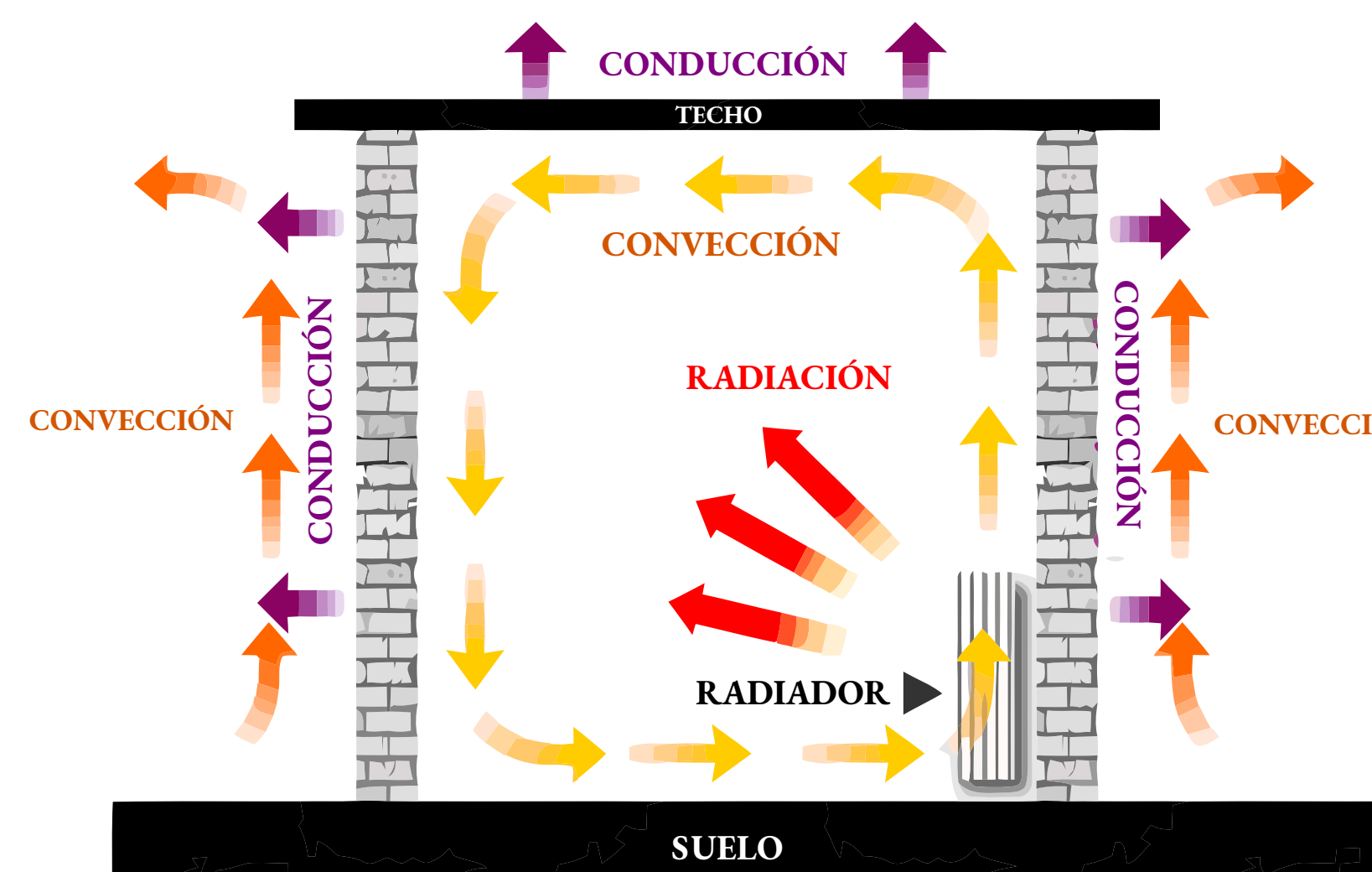
Adaptada de https://commons.wikimedia.org/wiki/File:M%C3%A9todos_de_transferencia_de_calor.svg .
