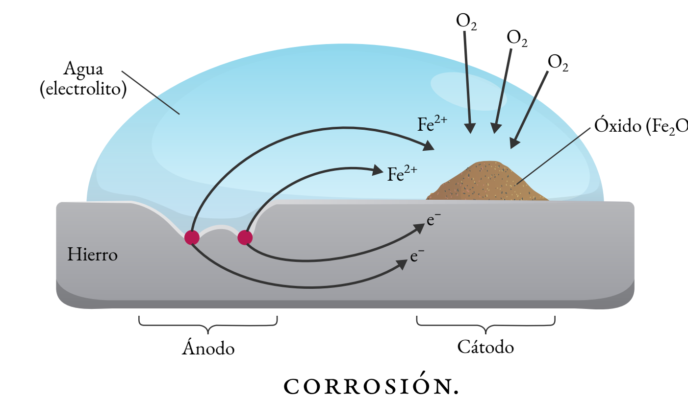
CORROSIÓN. Traducida y adaptada de https://www.coursehero.com/sg/general-chemistry/corrosion/ .
