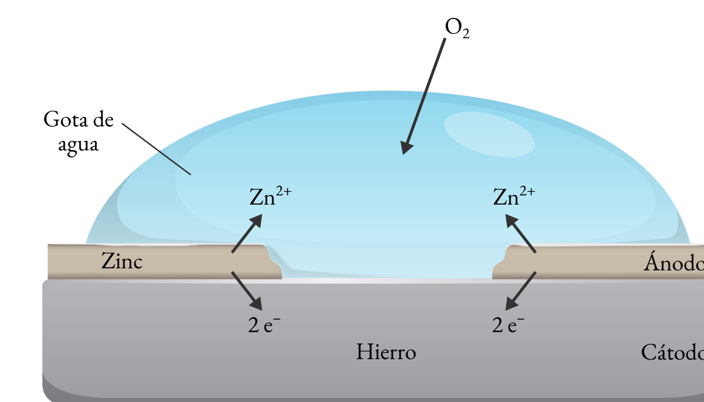
GALVANIZACIÓN. Traducida y adaptada de https://www.coursehero.com/sg/general-chemistry/corrosion/ .
